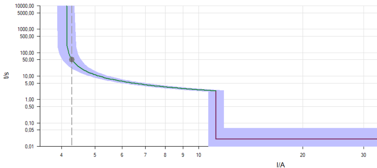
CURVA ANSI INVERSA LADO PRIMARIO (51P-1 ; 50P-1)
