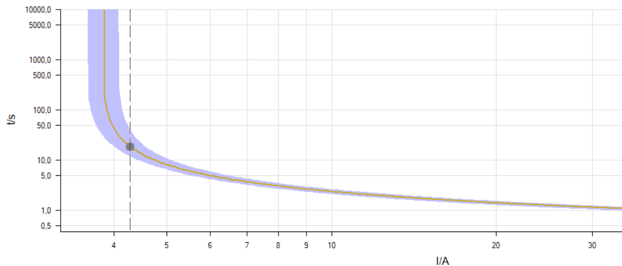
CURVA ANSI INVERSA LADO SECUNDARIO (51P-2)
