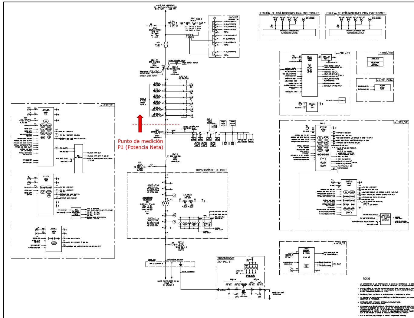
Gráfico 3. Esquema unilineal de la SE Tamarico 1 – parte 1.
