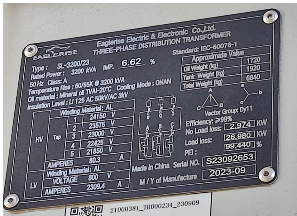
Figura 5-6: Foto de placa – Transformador principal
