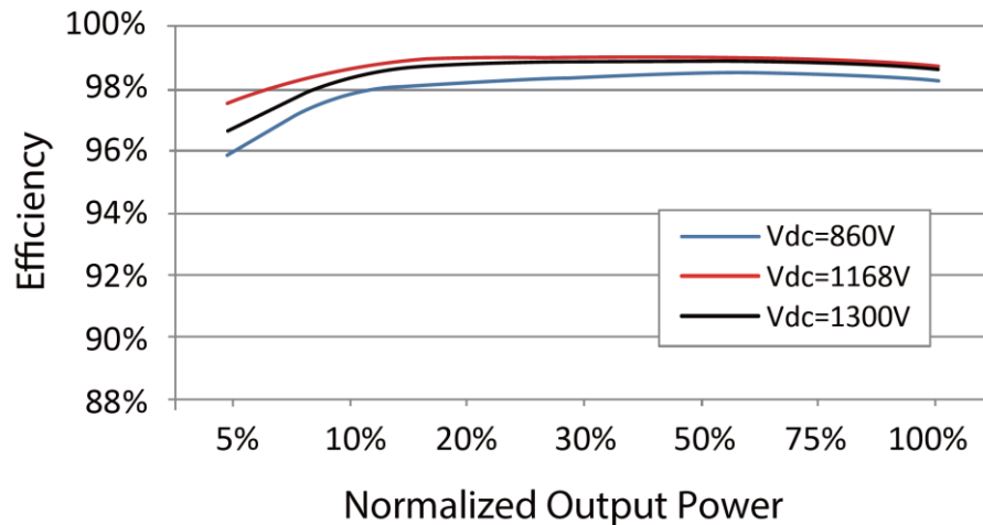
Figura 2-6: Curva de eficiencia – Inversores Sungrow SG350HX [5]
