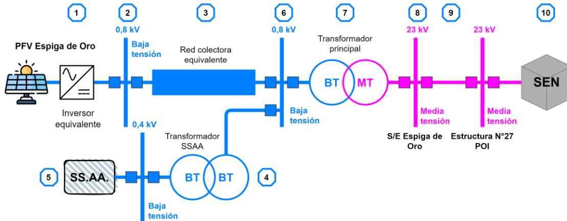
Figura 3-1: Esquema simplificado del PFV Espiga de Oro (NUP 3561)
