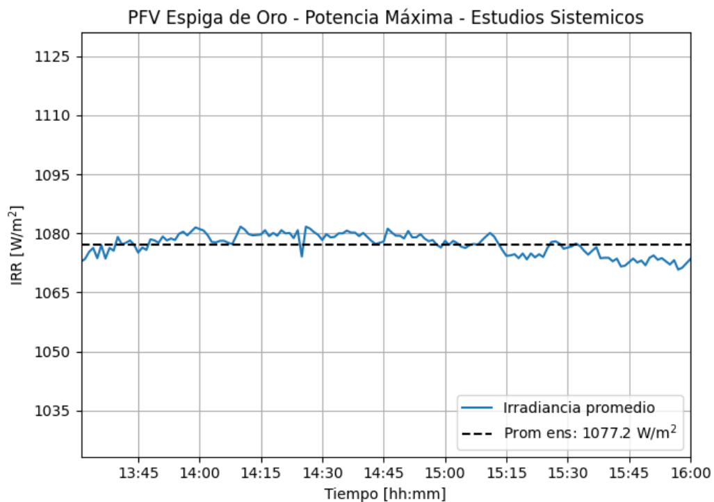
Figura 3-5: Irradiancia promedio del parque (IRR) – Ensayo de potencia máxima
