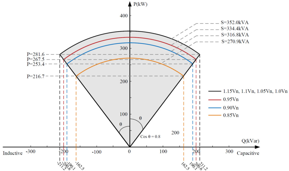
Figura 2-5: Curva de capacidad @30°C – Inversores Sungrow SG350HX [6]
