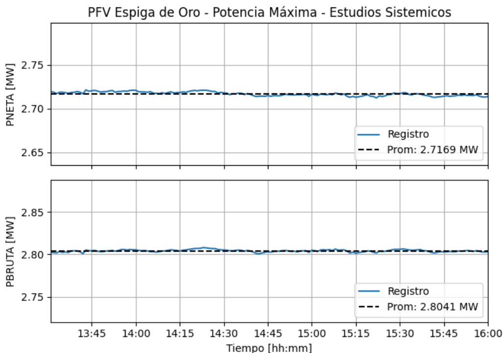
Figura 3-3: Potencia neta (PNETA) y Potencia bruta (PBRUTA) – Ensayo de potencia máxima
