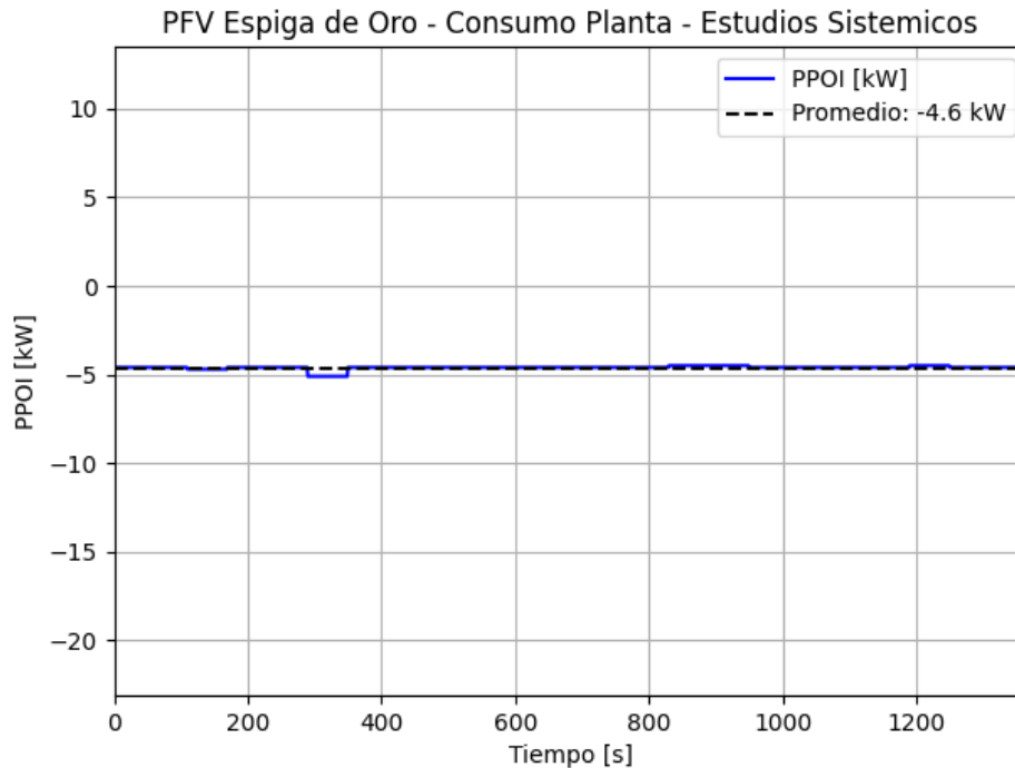
Figura 3-6: Potencia neta (P NETA ) - Ensayos para determinar el consumo de SSAA
