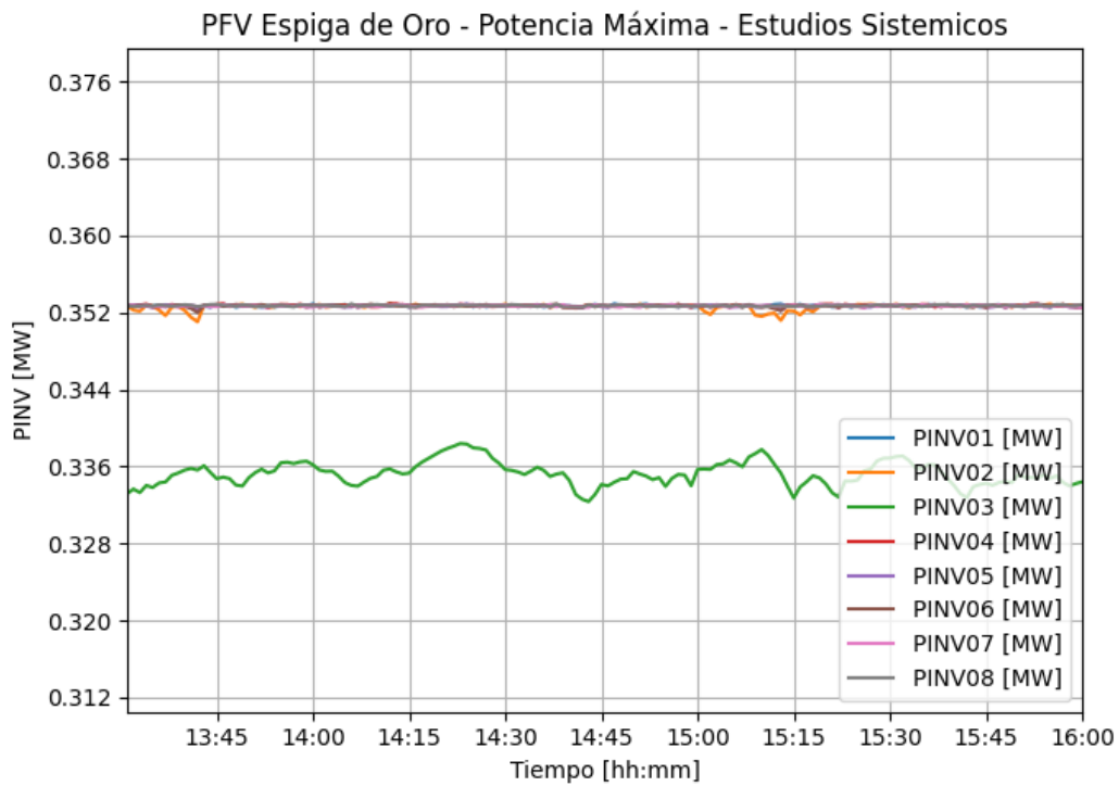
Figura 3-4: Potencia activa en bornes de los inversores (0,8 kV) (PINV) – Ensayo de potencia máxima
