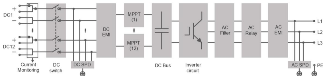
Figura 2-4: Diagrama de bloques simplificado – Inversores Sungrow SG350HX [5]
