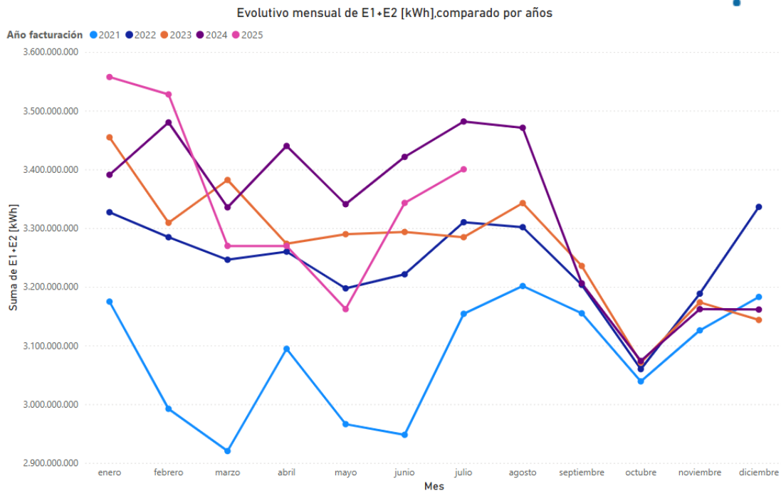
Figura 3: Evolutivo mensual de E1+E2 [kWh], comparado por años y mes de facturación
