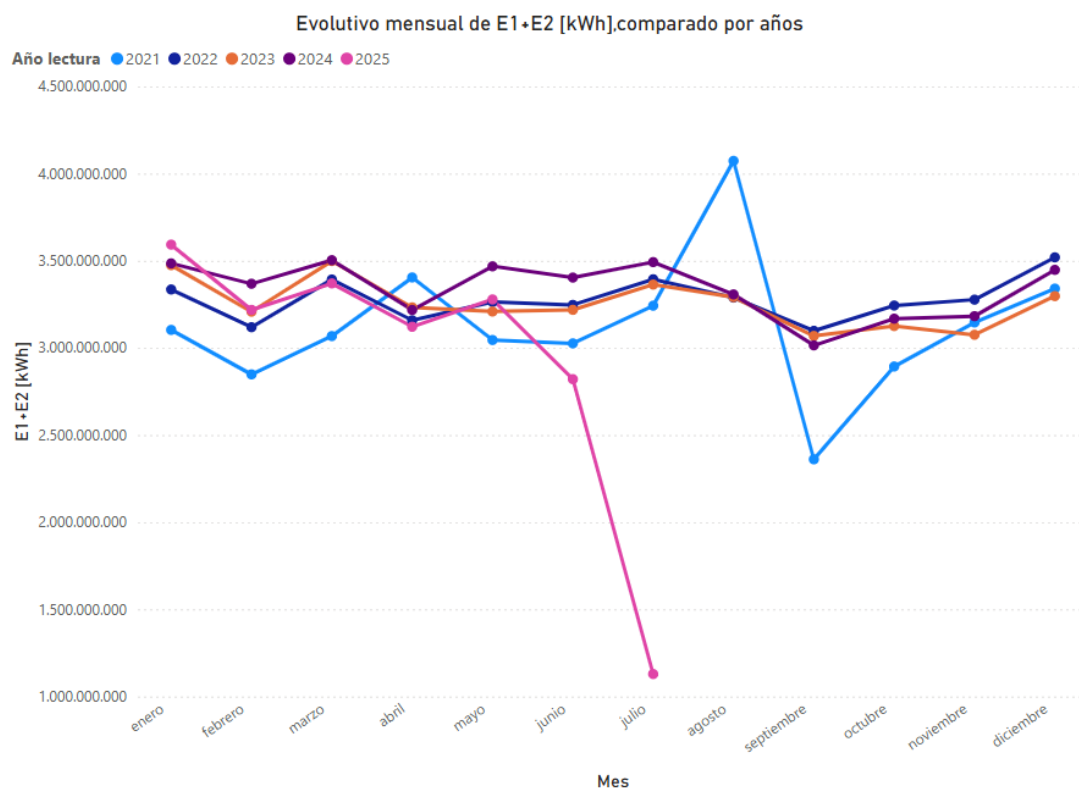
Figura 4: Evolutivo mensual de E1+E2 [kWh], comparado por años y mes de lectura
