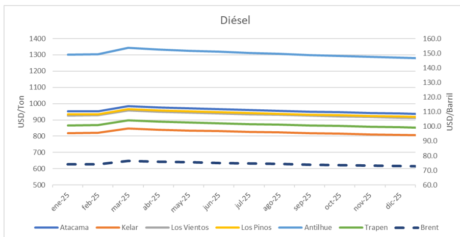
Figura 2. Costos de Diesel proyectados año 2025.
