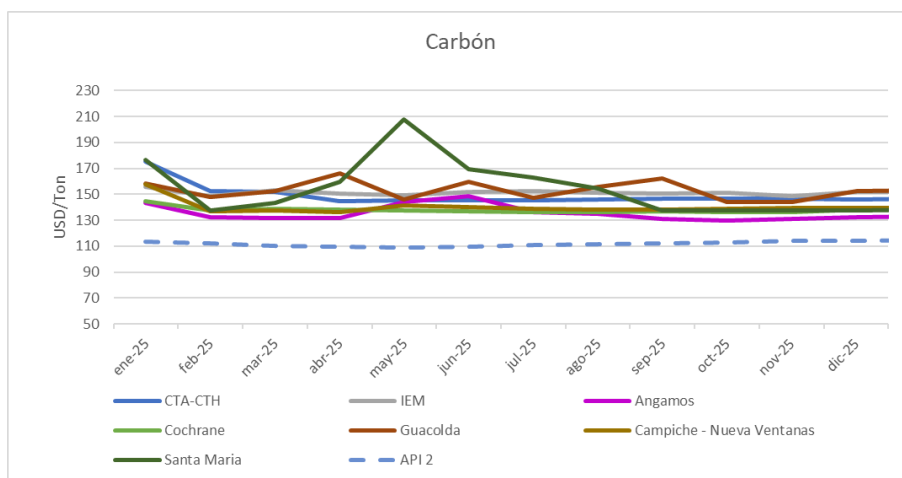
Figura 3. Costos de Carbón proyectados año 2025.
