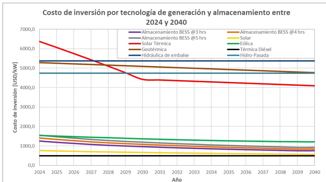
Gráfico 3: Proyección costos de inversión por tecnología de generación y almacenamiento
